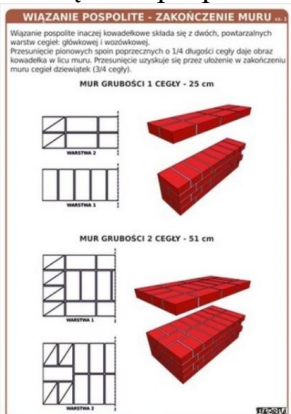
Wiązania pospolite - zakończenie muru cz. 3
