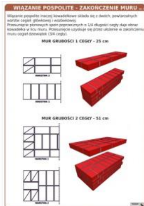
Wiązania pospolite cz. 1
