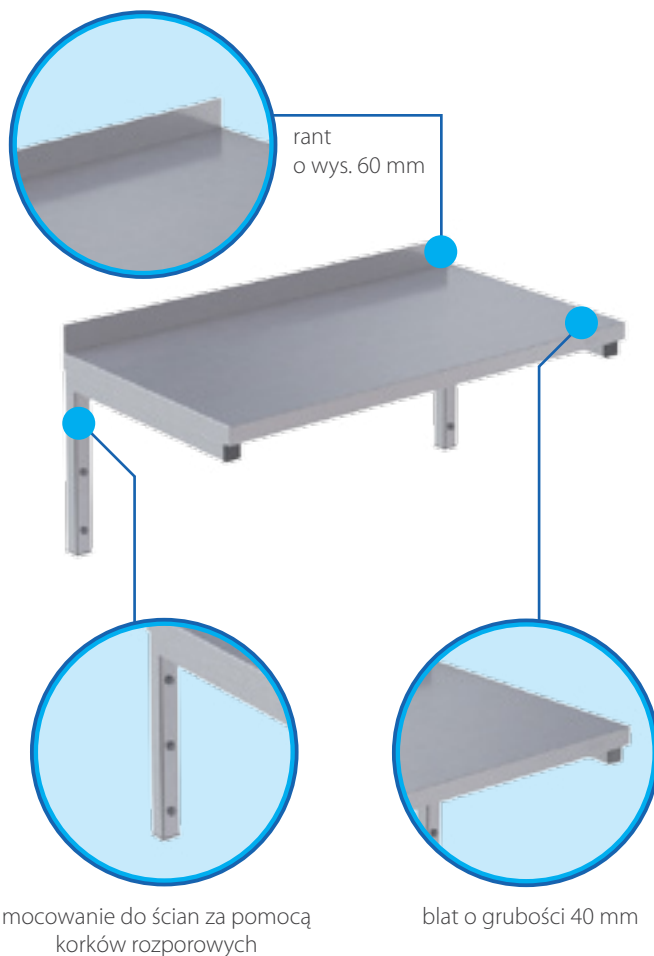
Blat mocowany do ściany z dwiema nogami
