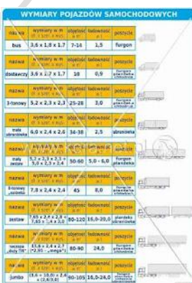
Wymiary pojazdów samochodowych
